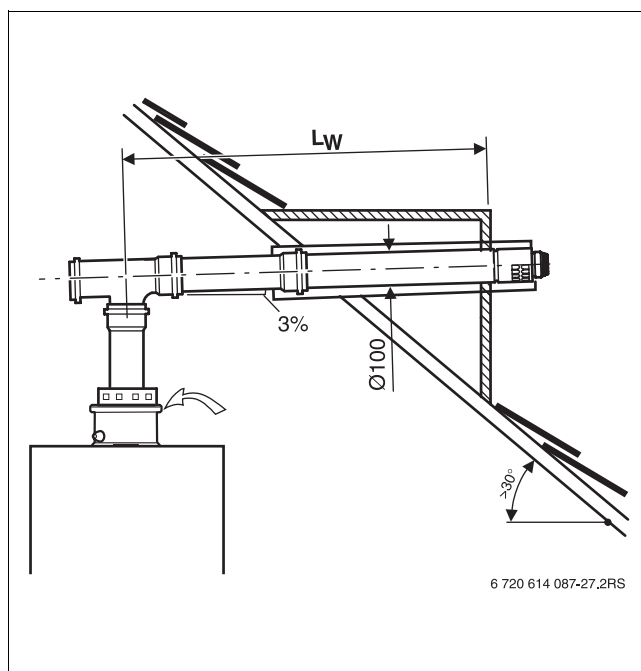
Рис 13 Одинарная труба через крышу (B 23 )
