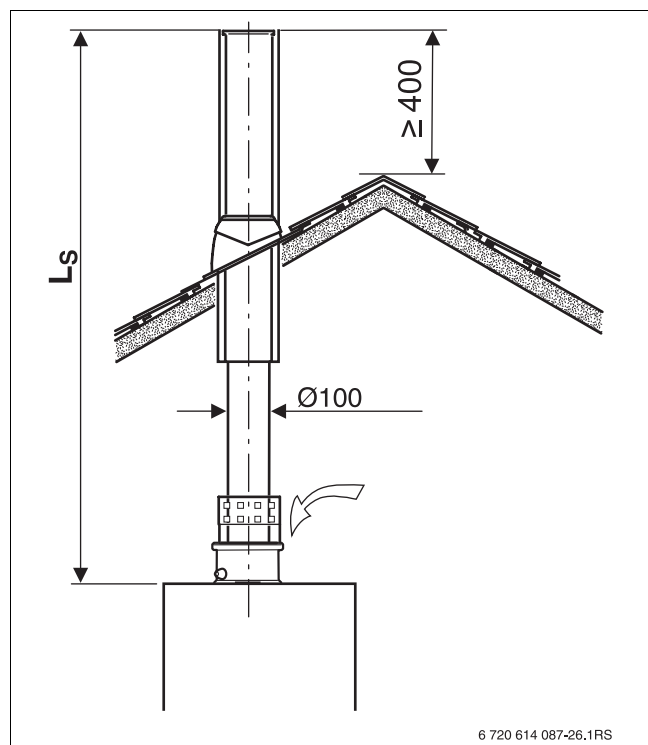
Рис 12 Одинарная труба через крышу (B 23 )
