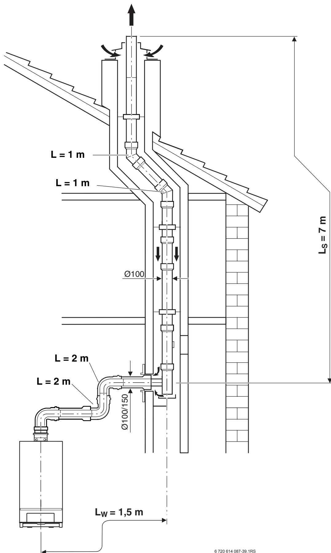
Рис 11 Пример определения длины дымовых труб
