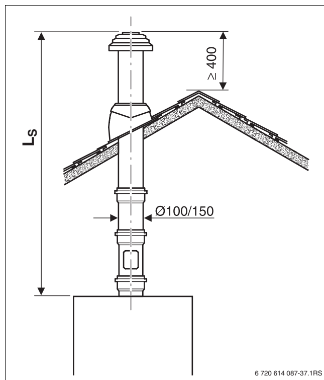
Рис 18 Вертикальная двойная труба ( C_{33(x)} )
