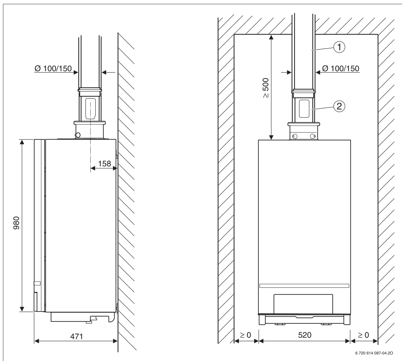
Рис 10 Монтажные размеры
