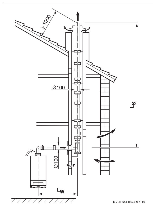
Рис 14 Одинарная труба в шахте ( B_{23} , жёсткая)
