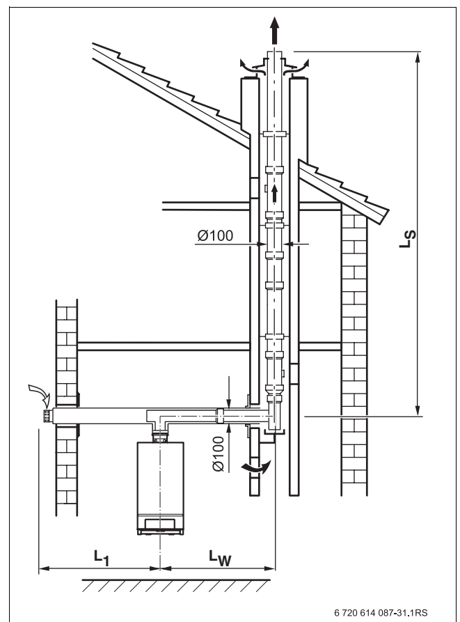
Рис 23 Раздельные трубы в шахте ( C_{83(x)} )
