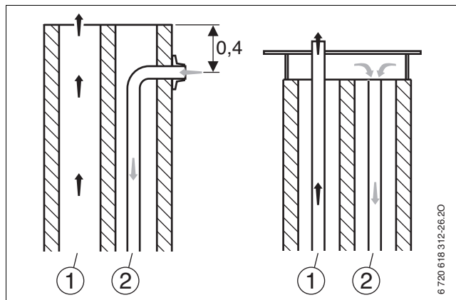
Рис 1 Примеры расположения устьев труб (размеры в м)
