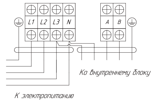
Клеммный терминал внешнего блока
