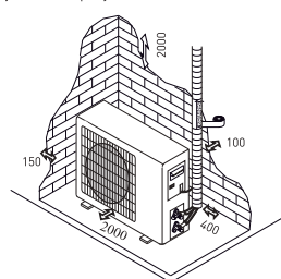
схема установки
