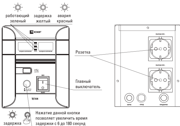
Рис. 3 Внешний вид стабилизатора F-1500-2000
