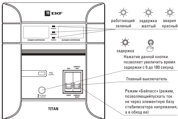
Рис. 4 Внешний вид стабилизатора F-3000-5000
