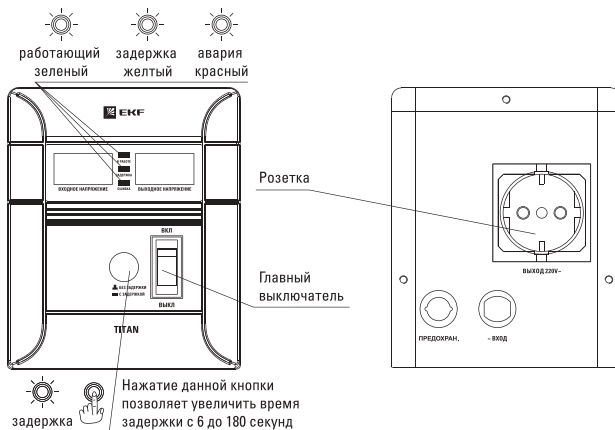
Рис. 2 Внешний вид стабилизатора F-500-1000
