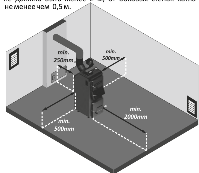
Рис 4. Расположение котла в котельной
