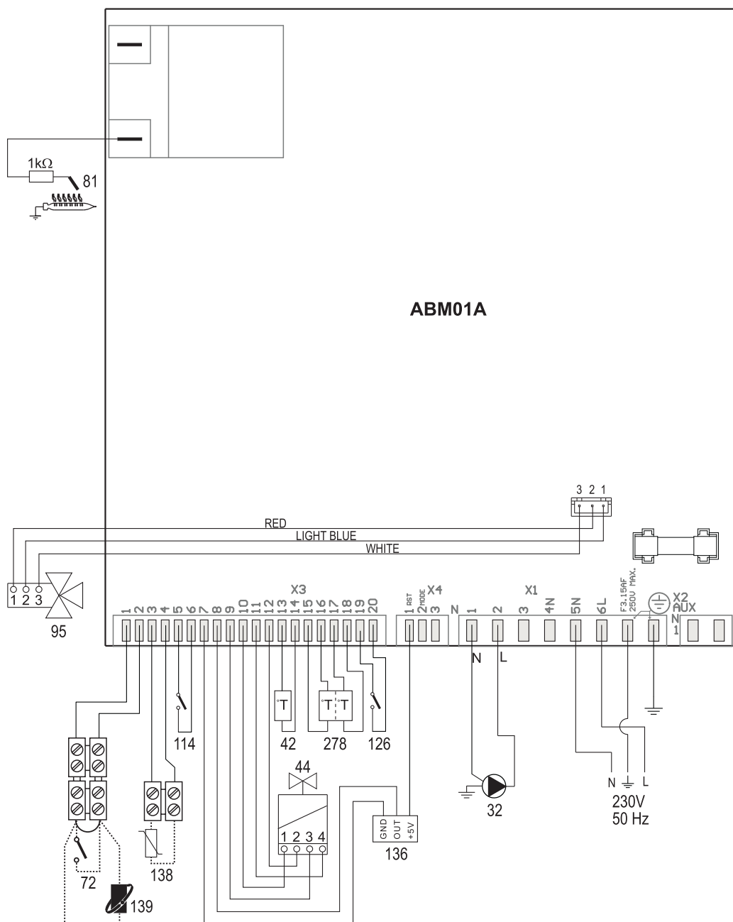
рис. 19- Электрическая схема
