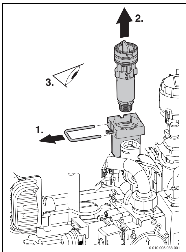
Рис. 30 Проверка фильтра в трубе холодной воды
