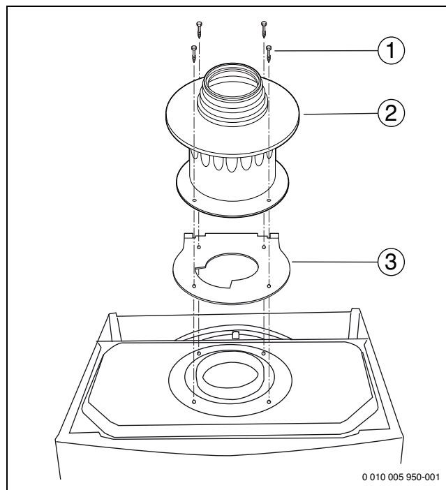
Рис. 15 При отводе дымовых газов B_{22} : установите адаптер и дроссельную диафрагму
