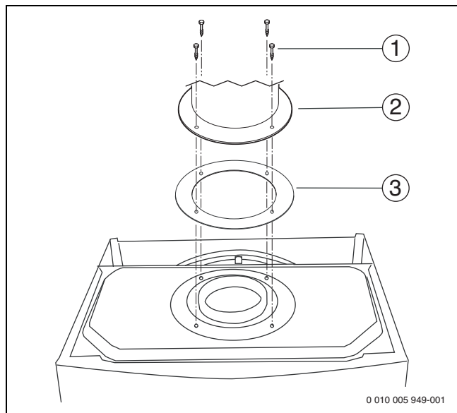
Рис. 14 Крепление переходника
