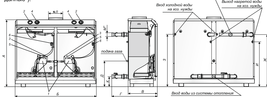
Рис. 2а. Схема конструкции котла "Житомир-3" модели КС-Г-080СН, КС-ГВ-080СН
