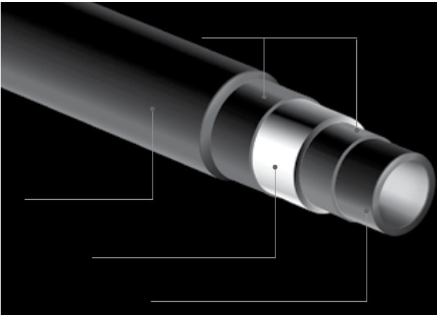
Рисунок 1. Структура трубы PE-Xb/Al/PE-Xb
