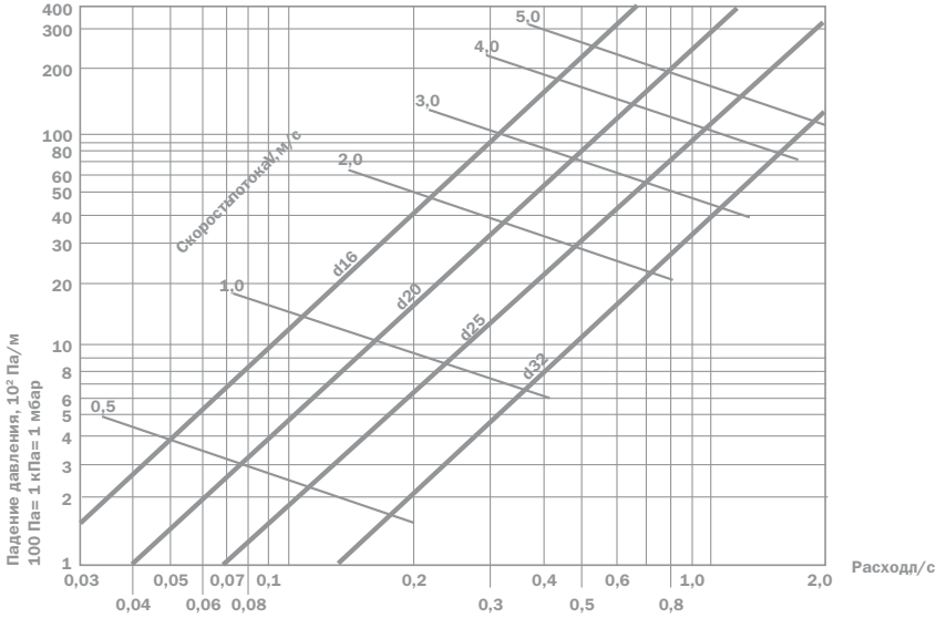
Рисунок 19. Номограмма потерь давления для труб PE-Xb/Al/PE-Xb в системе ГВС и ХВС.
