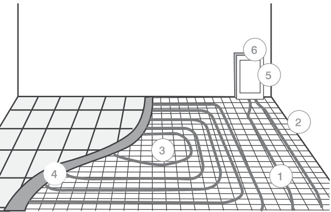
Рисунок 41. Схема системы напольного отопления: 1 - Трубы 2 - Изоляция стен 3 - Тепловая изоляция 4 - Монолитный пол 5 - Узел коллекторный 6 - Дверной порог
