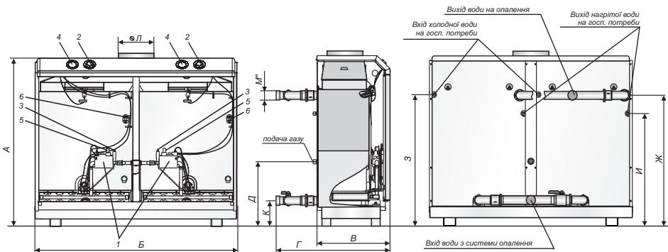
Мал. 2а. Схема конструкції котла "Житомир-3" моделі КС-Г-080СН, КС-ГВ-080СН
