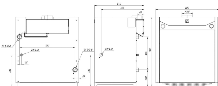
РИС 4. Lider Pro-600
