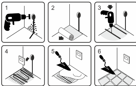
Рисунок 5 - Последовательность установки нагревательной секции.
