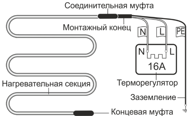
Рисунок 6 - Подключение теплого пола к терморегулятору.
