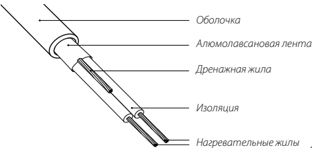
Конструкция двухжильного кабеля нагревательного WSS
