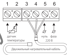
Схема подключения двужильной нагревательной секции WSS
