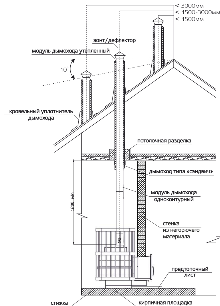
Схема устройства чугунной банной печи Kennet Атлант 22П сетка, ковка, панорама
