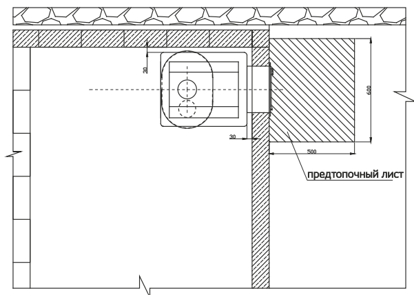
Рис. 4. Схема установки печи Kennet Атлант 22П сетка, ковка, панорама, вид сверху
